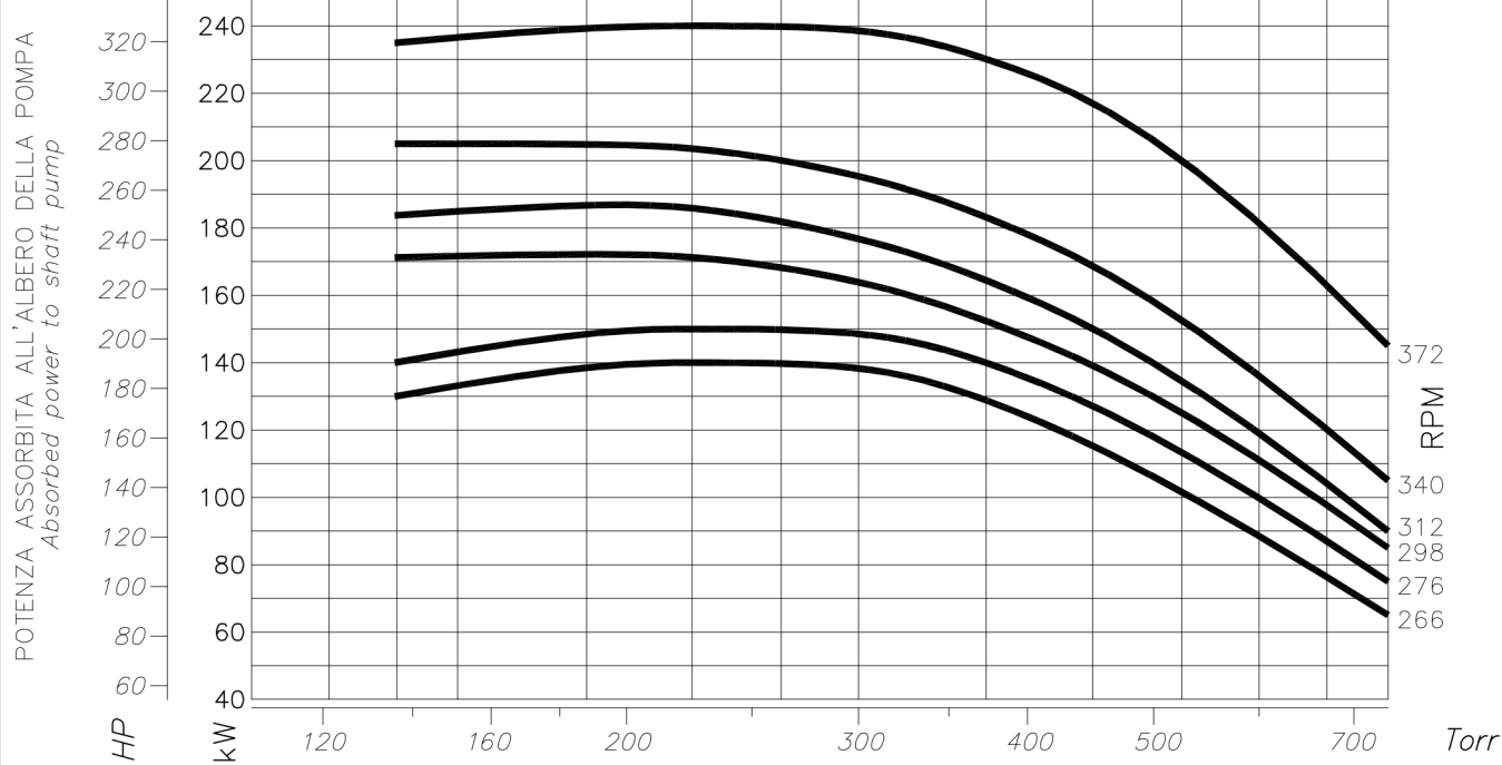
Liquido di servizio alle varie pressioni di aspirazione Service liquid at various inlet pressure
