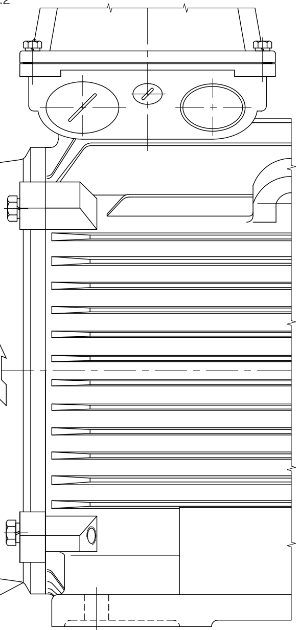
MOTORE TIPO 200L B35 Motor type 200L B35
